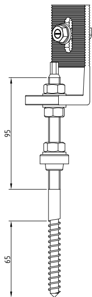
Sf.S. M10x200
