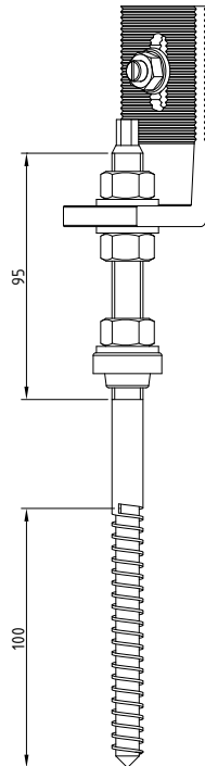
Sf.S. M12x250
