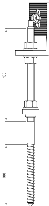
Sf.S. M12x300
