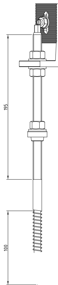
Sf.S. M12x350
