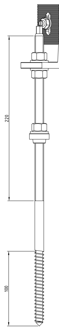
Sf.S. M12x400
