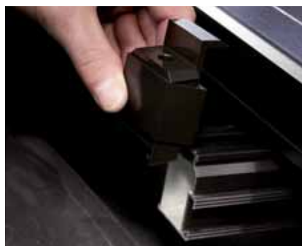
2 Inserire il morsetto terminale sulla guida di montaggio
