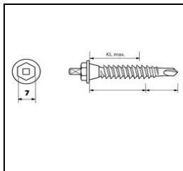
Bohrschraube SFS-SDK2-S-377- 6,0x35
