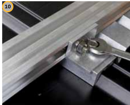
10 Installare le guide di montaggio con le squadrette
